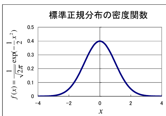
図 1 Excel グラフ
